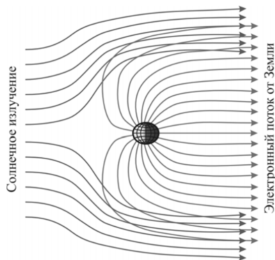
Рис. 5. Схема действия ионного потока Солнца на электронный поток Земли
