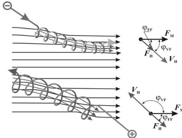
Рис. 1. Взаимодействие иона с магнитным полем
