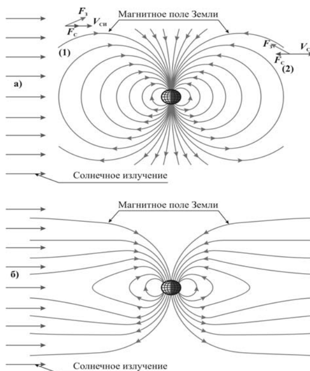
Рис. 4. При векторном суммировании магнитного поля Земли F_z и магнитного поля, создаваемого ионным потоком солнечного ветра F_c , и в области (1) и в области (2) (рис. а) магнитное поле Земли должно разворачиваться симметрично (рис. б)
