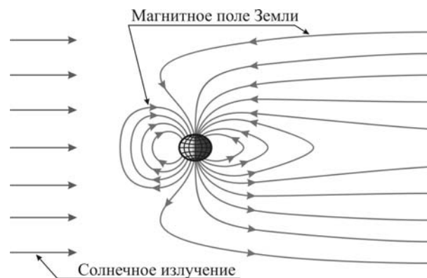
Рис. 3. Искажение магнитного поля Земли солнечным излучением
