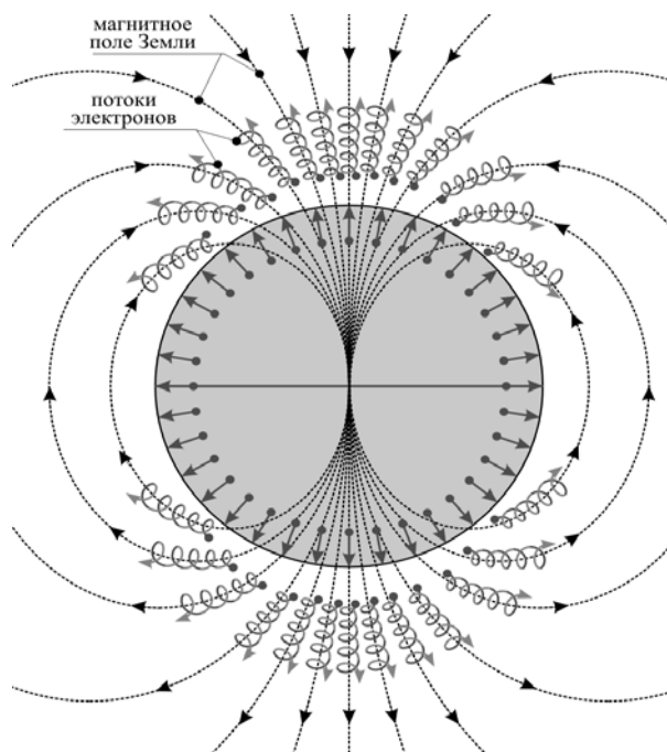
Рис. 2. Схема преобразования электрической энергии электронных потоков в энергию магнитного поля Земли
