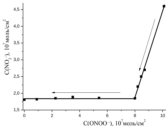
Рис. 3. Изменение концентраций \text{ONOO}^- и \text{NO}_2^- в процессе фотоотжига (ДРТ-1000, фильтр \lambda \geq 310 нм) \text{KNO}_3 , фотолитизированного светом 253.7 нм (4 час)
