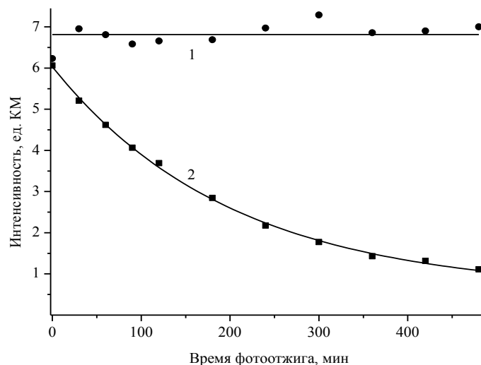
Рис. 1. Кинетика фотоотбеливания полос, соответствующих \text{ONOO}^- ( 940\text{ см}^{-1} (2)) и \text{NO}_2^- ( 1250\text{ см}^{-1} (1)) в фотолизированном \text{KNO}_3 , с коррекцией на термические пост-процессы. Время предварительного фотолиза 70 мин.
