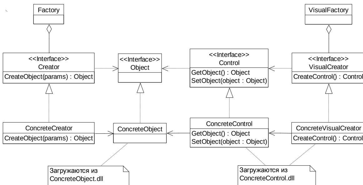
Рис. 1. Общая архитектура подсистемы подключаемых модулей
