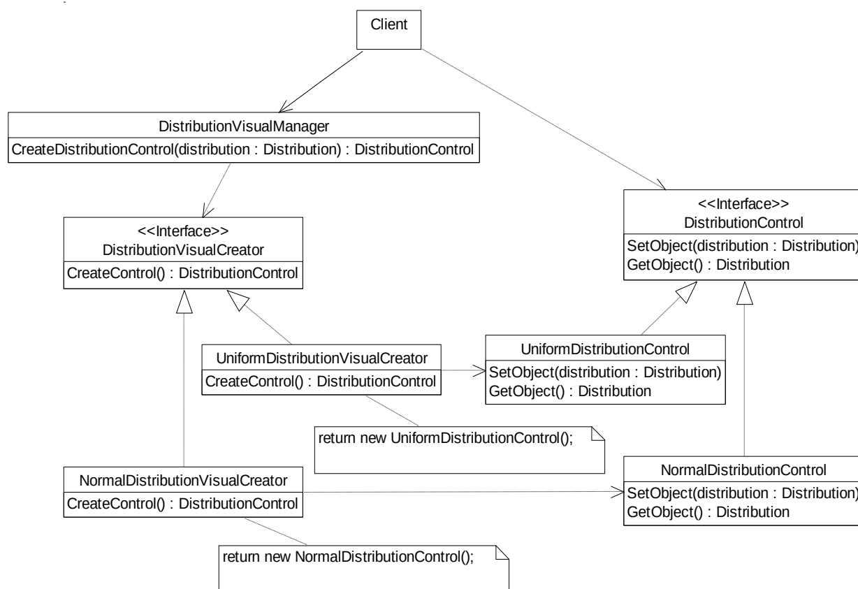
Рис. 4. Реализация визуального представления объектов-распределений случайных величин
