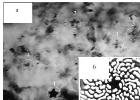
Рис. 3. Образование звездочек в точках выхода оси L_5 на электронно-микроскопических снимках ПНБ (а) и при укладе светлых блоков в самоорганизующейся структуре (б); 1, 2, 3, 4, 5 – разные уровни проявления звездочек
