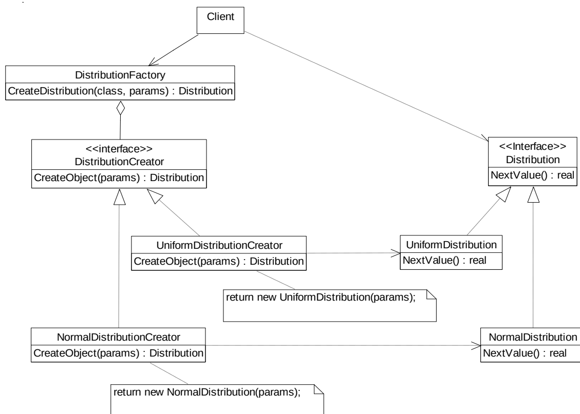
Рис. 3. Реализация подхода для объектов-распределений случайных величин
