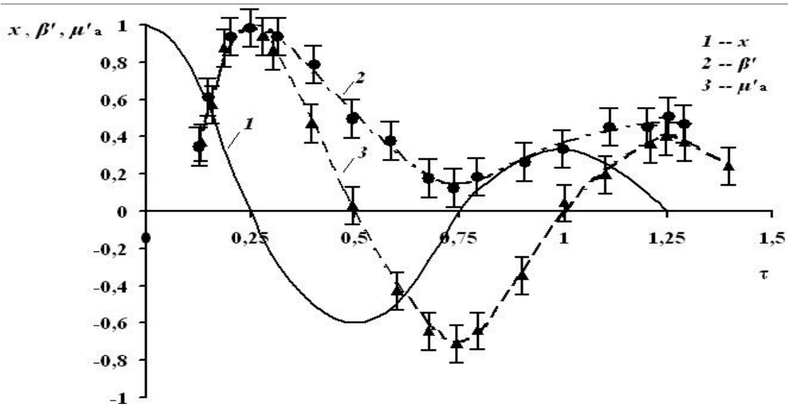
Рис. 1. Зависимость смещения иона x в облаке Коттрелла относительно линии дислокации; относительно удержанного объёма \beta' = \beta / \beta_{\max} ; амбипольной дрейфовой подвижности \mu'_a = \mu_a / \mu_{a,\max}
