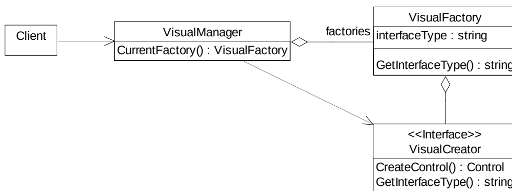
Рис. 2. Управление динамическим подключением фабрик визуальных элементов
