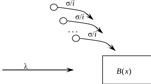
Рис. 1. Немарковская динамическая RQ-система с конфликтами заявок
