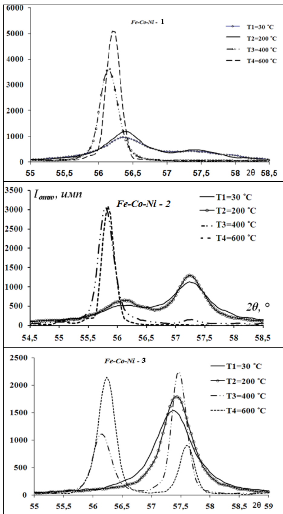
Рис. 2. Дифрактограммы НСП Fe-Co-Ni
