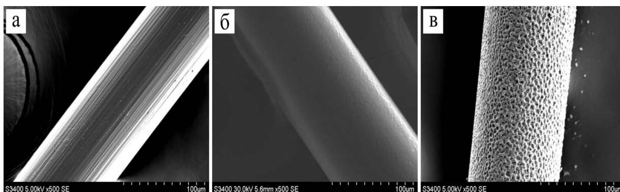
Рис. 5. Сканирующая электронная микроскопия поверхности шовного материала: а – немодифицированная нить; б – нить + ПГБВ; в – нить + ПГБВ + модифицирующий слой + гепарин. Увеличение – 500 раз
