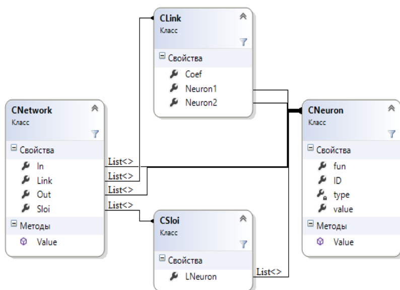
Рис. 7. Диаграмма классов
