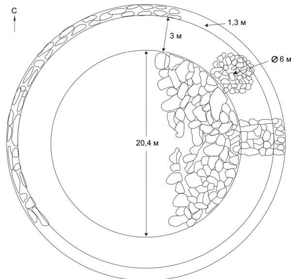
Рис. 1. План кургана с изваянием. Бесоба. Схематический рисунок М. К. Кадырбаева
