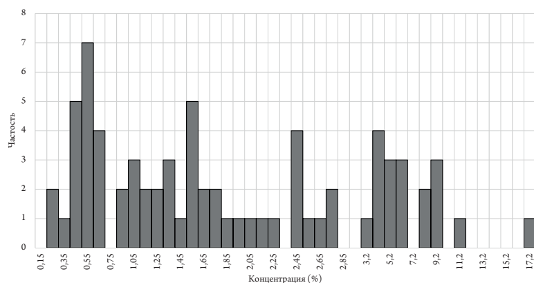
Рис. 3. Гистограмма распределения примесей мышьяка в металле предметов из погребений лепешкинского этапа тагарской культуры могильника Серебряково I Fig. 3. Arsenic impurities in the metal of artifacts from the burials of Lepeshkinsky Stage, Serebryakovo I
