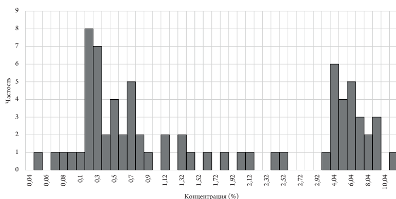
Рис. 2. Гистограмма распределения примесей олова в металле предметов из погребений лепешкинского этапа тагарской культуры могильника Серебряково I Fig. 2. Tin impurities in the metal artifacts from the burials of Lepeshkinsky Stage, Serebryakovo I
