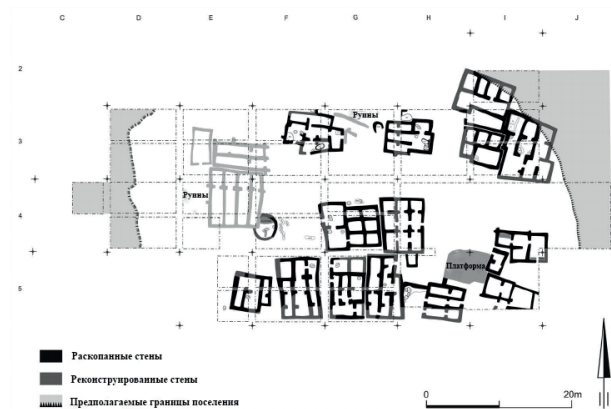
Рис. 5. Телль Саби Абьяд I, раскоп III: план здания в слое A4, датированном радиоуглеродным методом, ок. 6430–6395 гг. до н. э. [4, р. 37]
